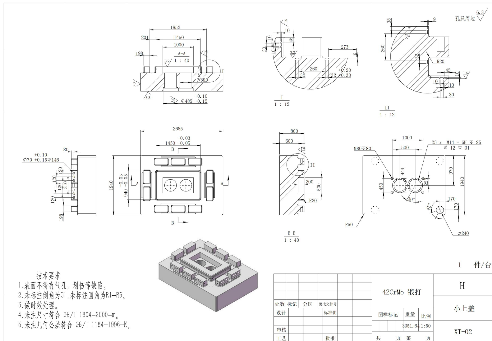
图3 箱体上盖图纸
