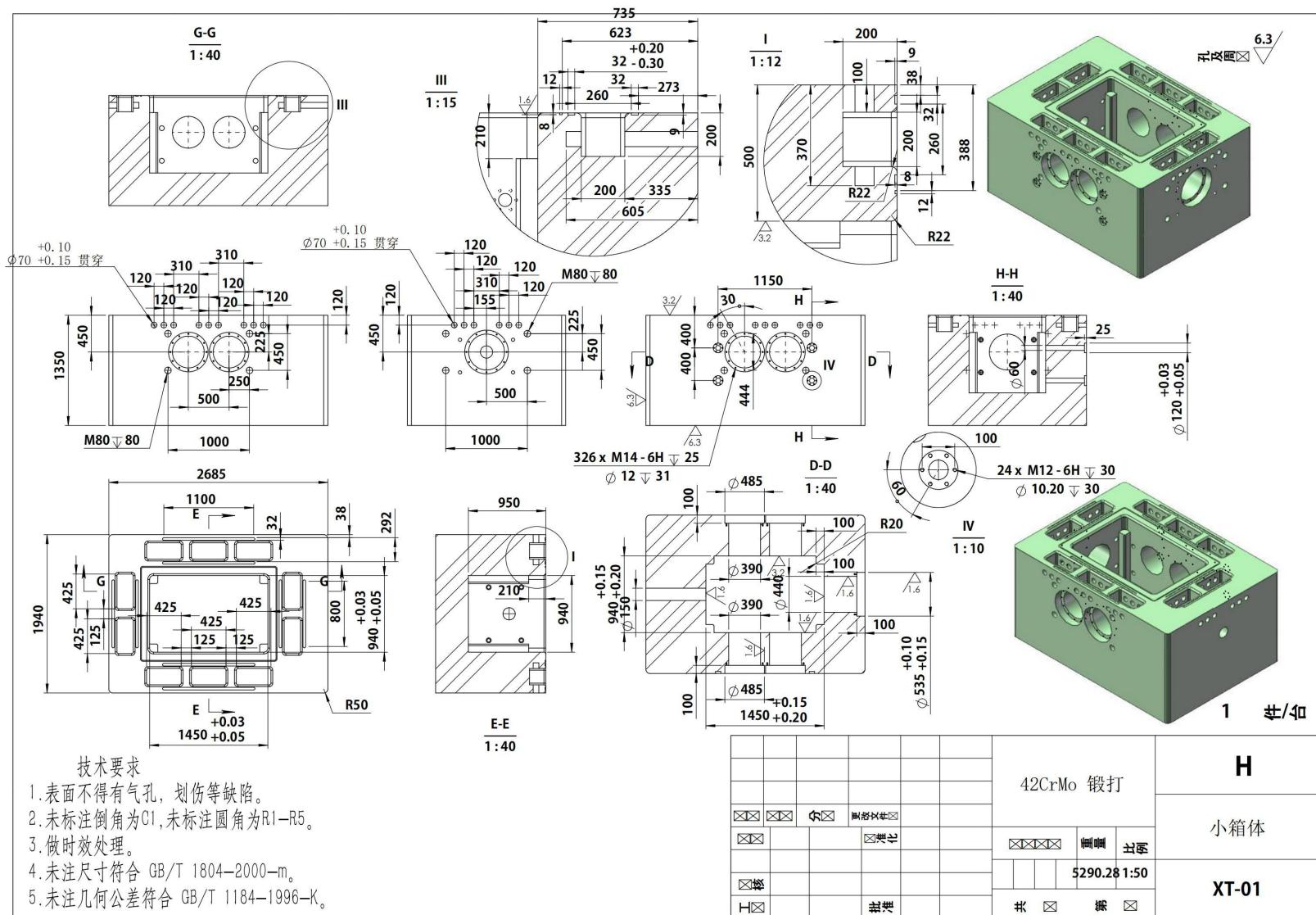
图2 箱体主体图纸
